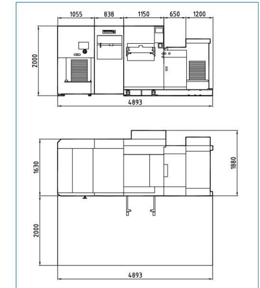
JY-76E Floor Plan
