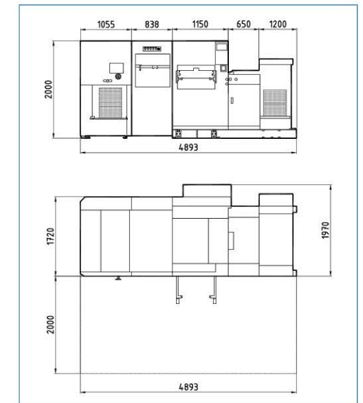
JY-85E Floor Plan
